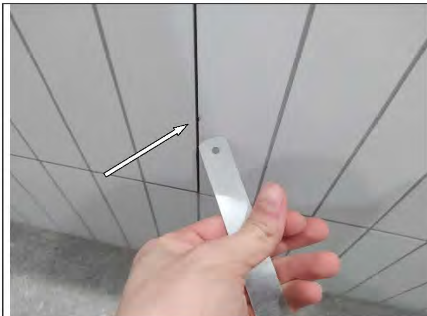
Фото №31. Отбитости настенной керамической плитки в ванной комнате
