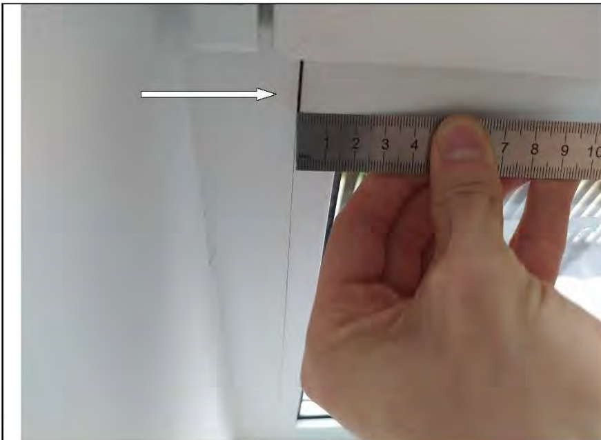
Фото №16. Профиль ПВХ оконного блока в спальне имеет дефекты (зазор).
