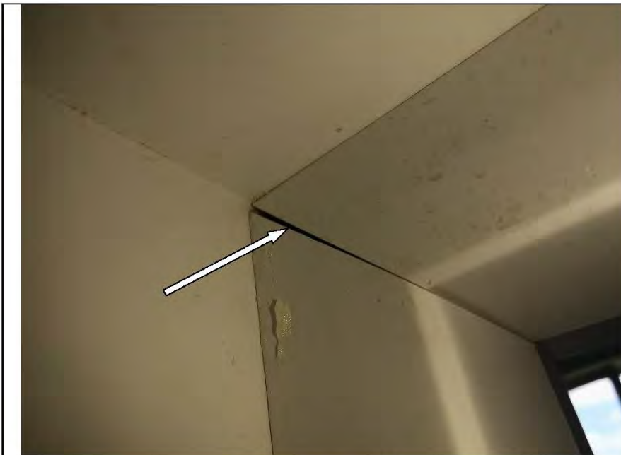
Фото №55. Ненадежное соединение элементов деревянного дверного блока (коробки) в спальне.
