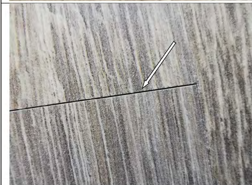
Фото №27. Неполное заполнение шовного пространства напольной керамической плитки в коридоре.
