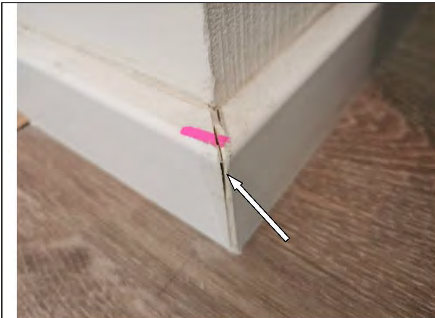
Фото №28. Деревянные напольные плинтуса имеют зазор более 0,3 мм в месте соединения элементов в коридоре.
