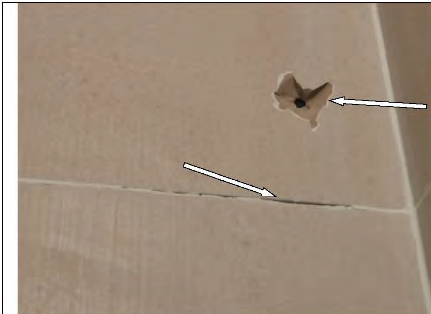
Фото №19. Неравномерное заполнение шва настенной керамической плитки затиروчным составом, отбитость настенной керамической плитки в ванной комнате.
