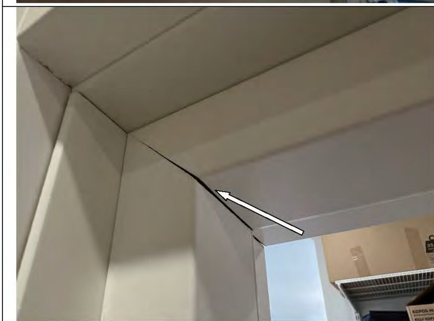
Фото №93. Элементы дверного блока в ванной комнате соединены не надежно.
