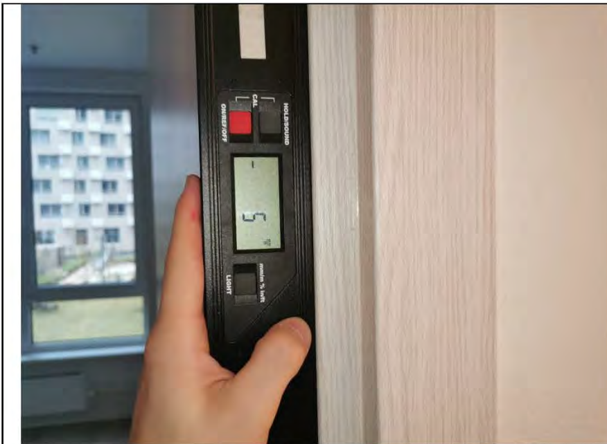
Фото №58. Отклонение коробки деревянного дверного блока от уровня вертикальности в спальне.
