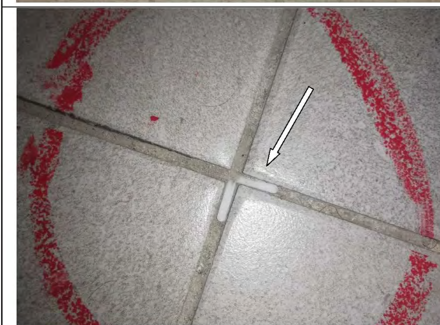
Фото №36. Затирка напольной керамической плитки в ванной комнате выполнена с нарушениями.
