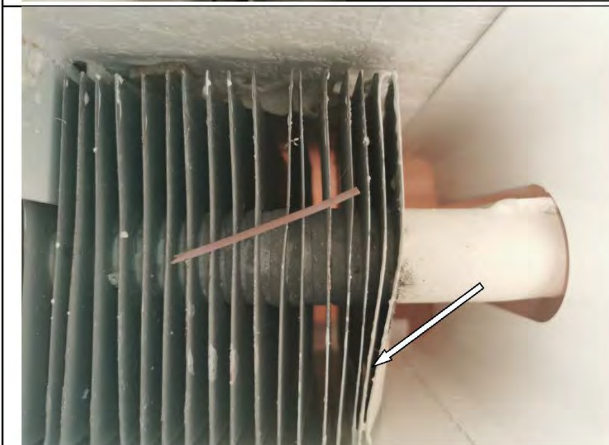
Фото №71. Замятие сот радиатора в кухне.
