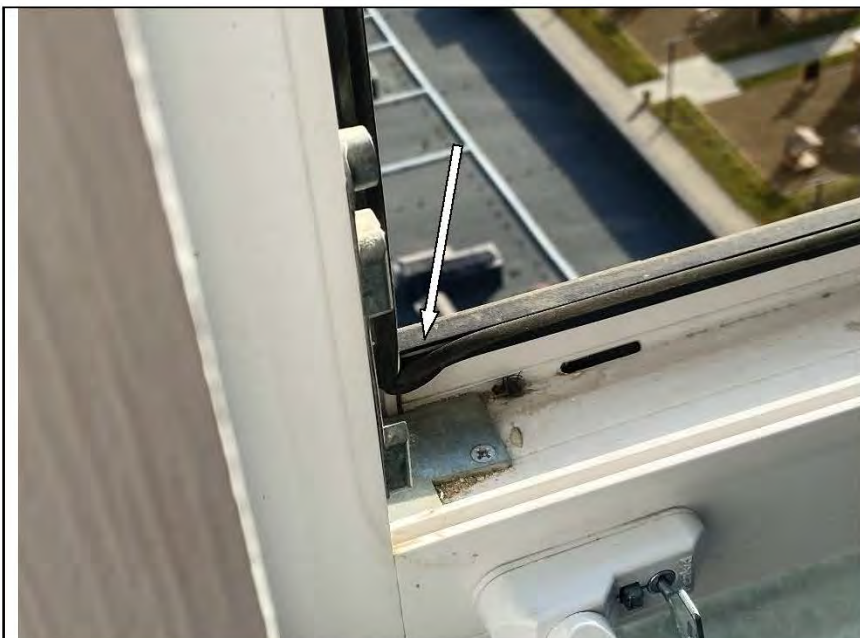
Фото №100. Дефект на уплотнительной ленте оконного блока ПВХ в спальне.
