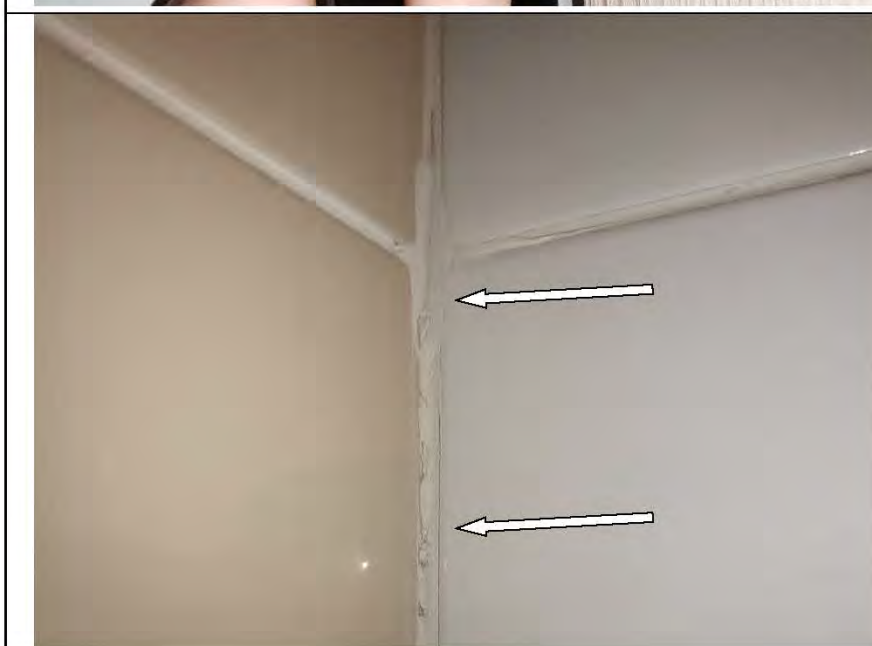
Фото №39. Неравномерное заполнение шовного пространства настенной керамической плитки затиروчным составом в санузле.
