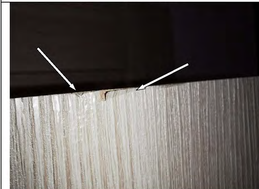
Фото №122. Повреждение ламинации на полотне деревянного дверного блока в кухне.
