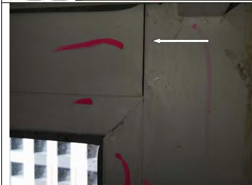
Фото №81. Зазор в месте стыка профилей ПВХ оконного блока в кухне.
