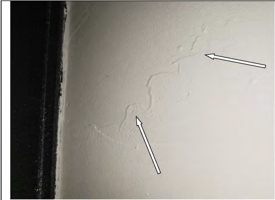
Фото №133. Окрашенные откосы входного дверного блока выполнены с дефектами.
