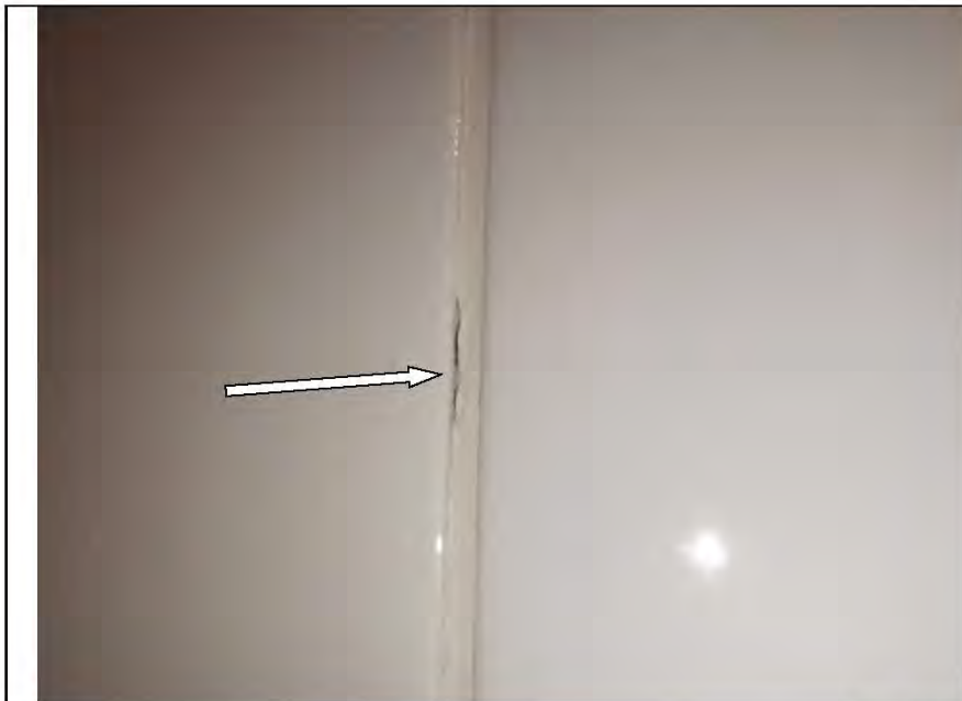
Фото №40. Неравномерное заполнение шовного пространства настенной керамической плитки затирочным составом в санузле.
