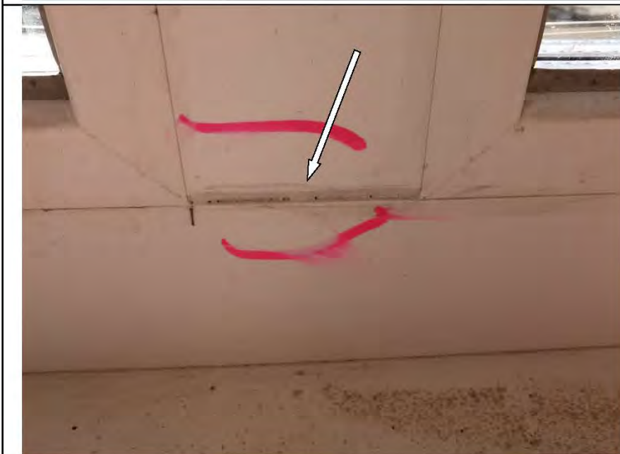
Фото №86. Зазор в месте стыка профилей ПВХ оконного блока в детской.
