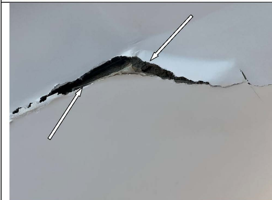
Фото №11. Разрушение конструкции подвесного потолка в спальне.
