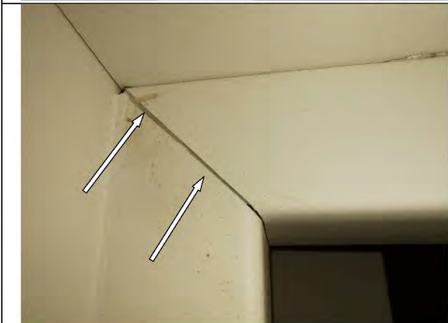
Фото №53. Элементы дверного блока (коробка) соединены не надежно в ванной комнате.
