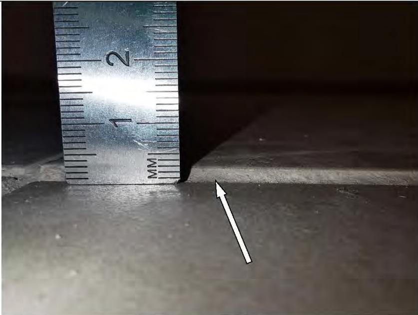
Фото №28. Уступы керамической плитки пола в коридоре.
