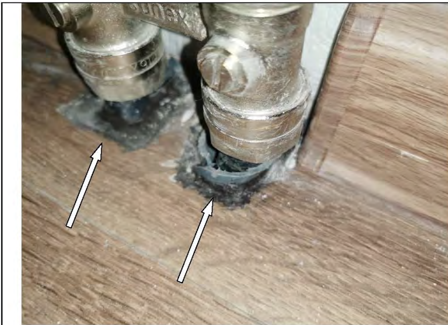
Фото №22. Заделка отверстия для трубопровода отопления в напольном покрытии из ламината выполнена с дефектом на кухне.
