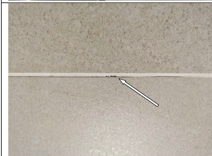
Фото №20. Неравномерное заполнение шовного пространства настенной керамической плитки затирочным составом в ванной комнате.
