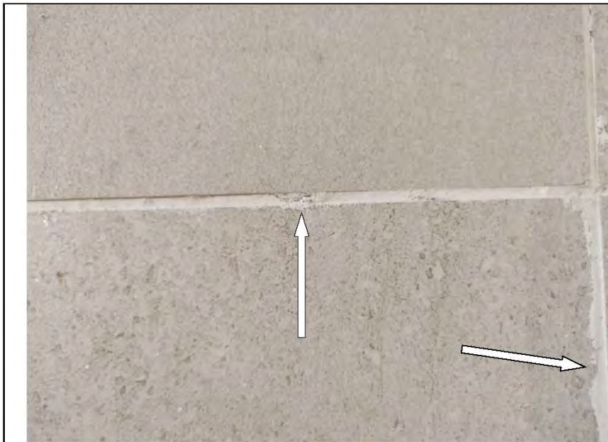
Фото №28. Неравномерное заполнение шовного пространства напольной керамической плитки затиروчным составом в коридоре.
