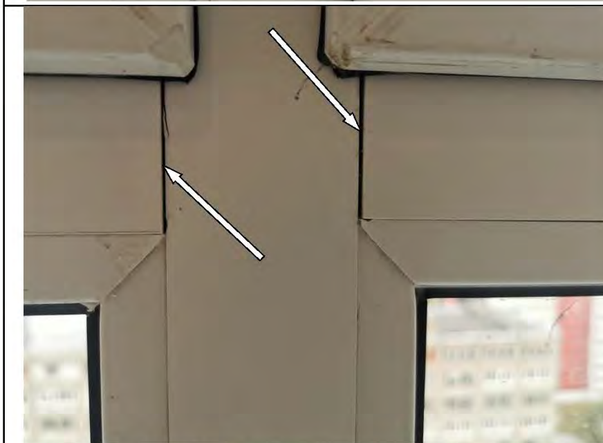
Фото №38. Зазоры в месте стыка профилей ПВХ оконного блока в кухне.
