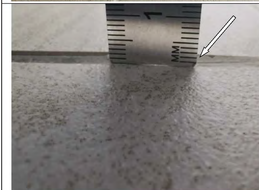
Фото №30. Уступы керамической плитки пола в коридоре.
