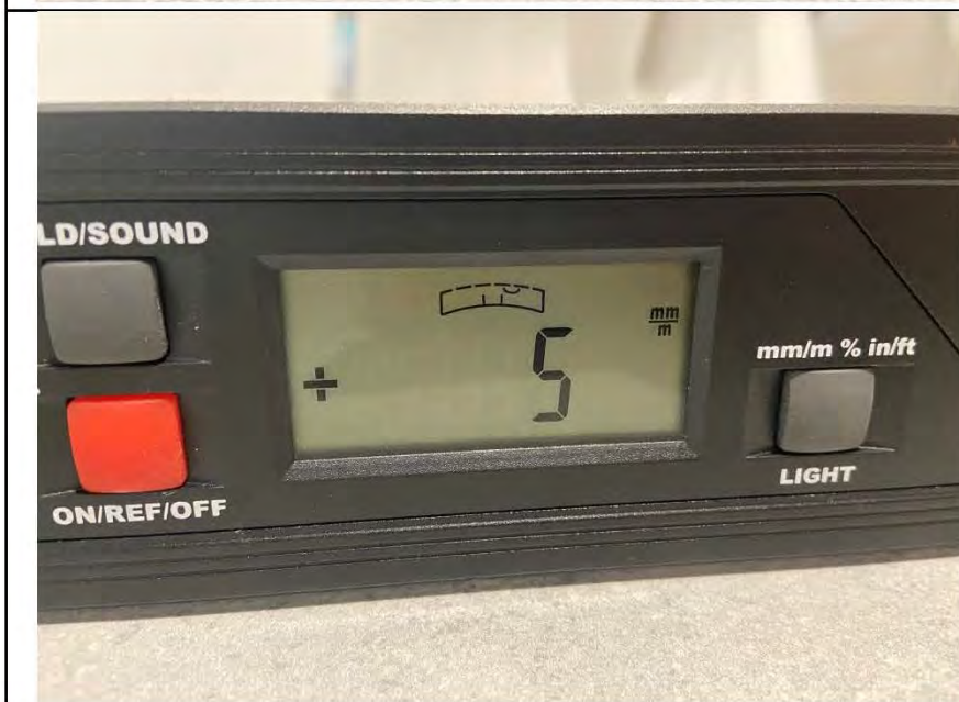
Фото №18. Отклонения поверхности напольного покрытия из керамической плитки в ванной комнате.
