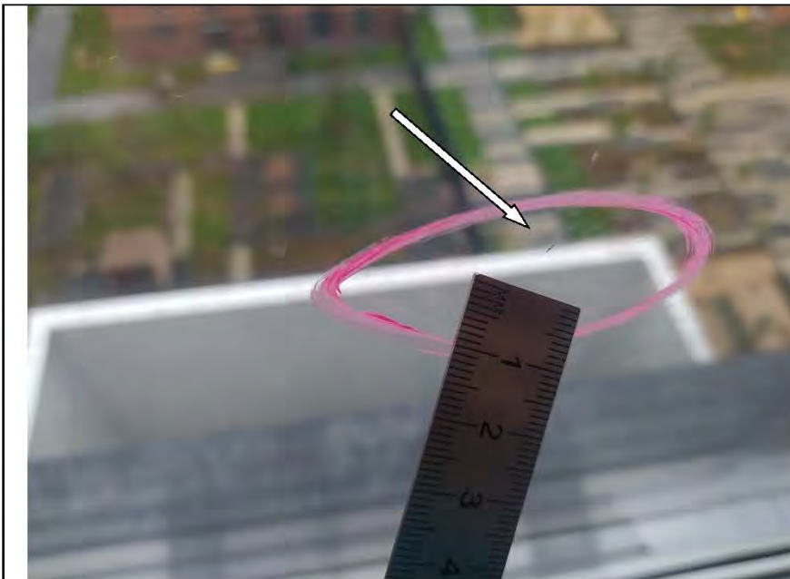
Фото №25. На стеклопакете оконного блока ПВХ в спальне имеется дефект (окалина).
