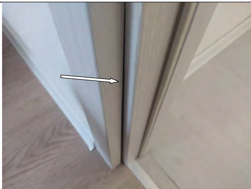
Фото №35. Коробка дверного блока в спальне не закреплена к проему.
