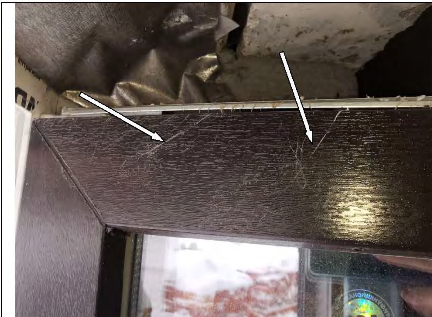
Фото №13. Царапины на профиле ПВХ оконного блока.
