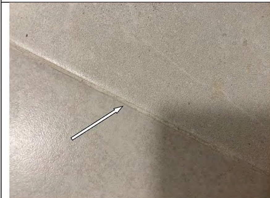
Фото №29. Неровные швы напольной керамической плитки в ванной комнате.
