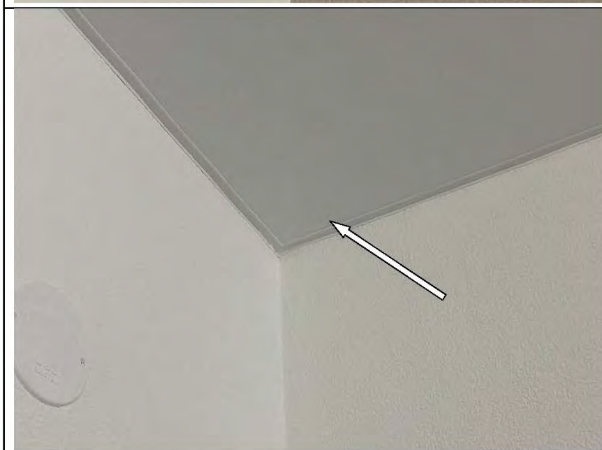
Фото №81. Дефект на поверхности натяжного потолка в детской.
