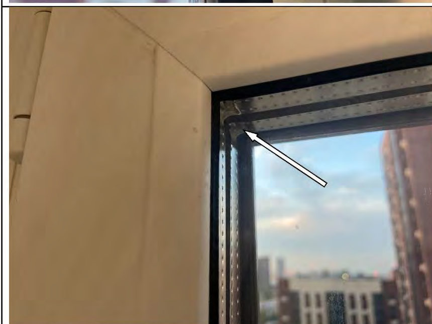
Фото №59. Дефект на уплотнительной ленте оконного блока ПВХ в спальне.
