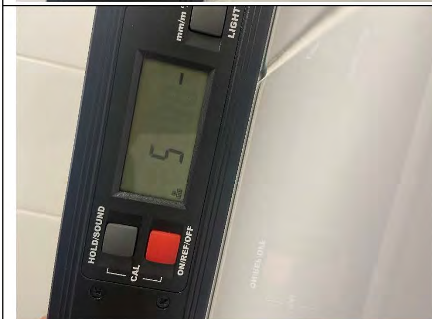
Фото №8. Отклонения поверхности стен от вертикали в ванной комнате.
