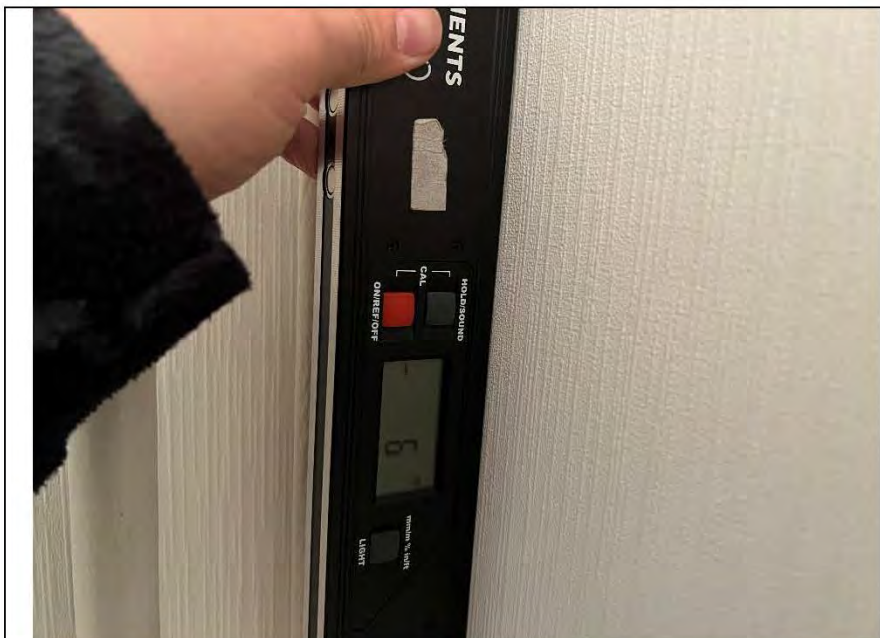
Фото №10. Измерение уровня стен в гостиной.
