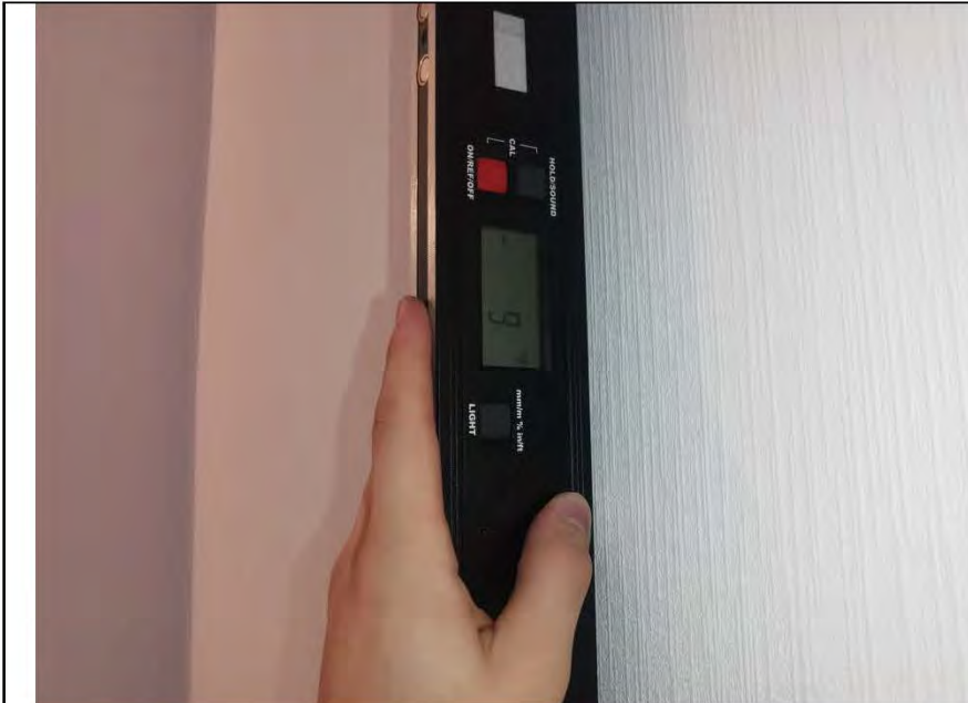
Фото №10. Измерение уровня стен в кухне.
