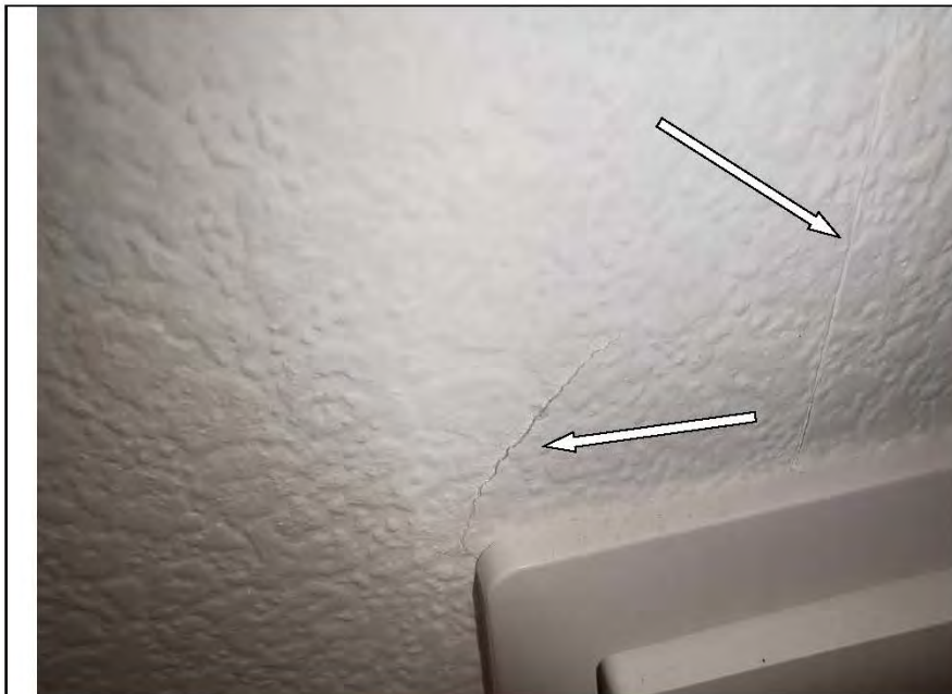
Фото №19. Разрыв обойного полотна и читаемые обойные стыки в прихожей
