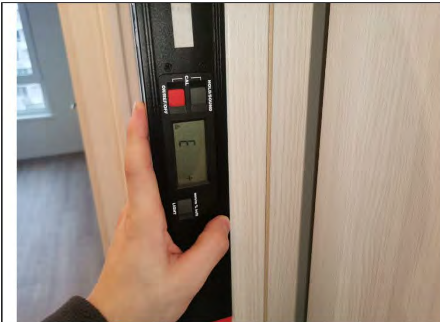
Фото №106. Отклонение коробки деревянного дверного блока от уровня вертикальности в детской.
