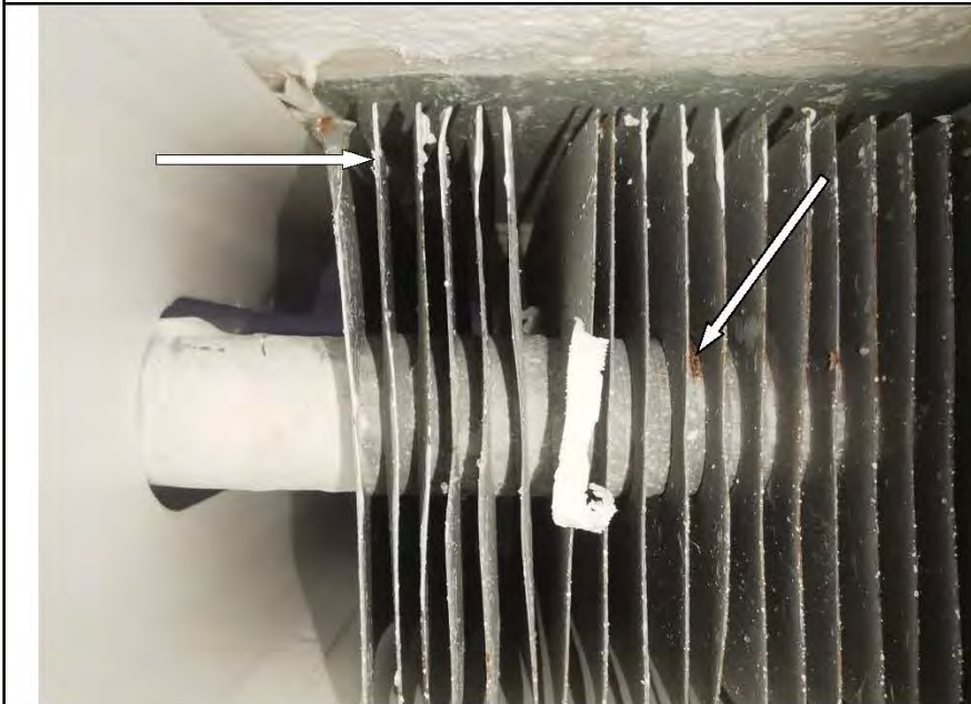
Фото №132. Замытие и коррозия радиатора в гостиной.
