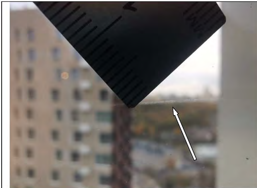
Фото №88. Царапины на стеклопакете оконного блока ПВХ в кухне.
