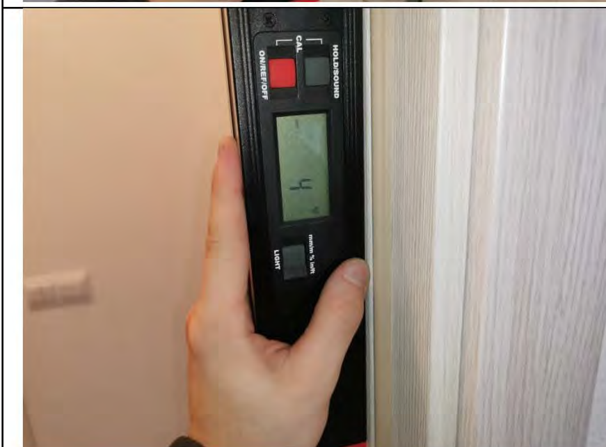
Фото №107. Отклонение коробки деревянного дверного блока от уровня вертикальности в гостиной.
