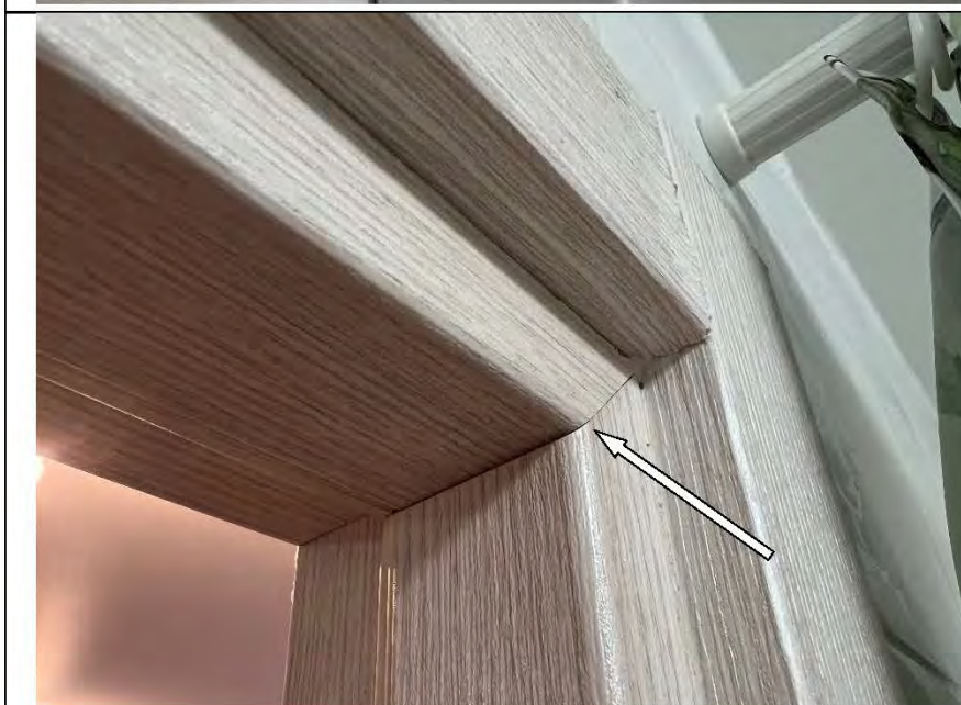
Фото №44. Элементы дверного блока соединены не надежно в ванной комнате.
