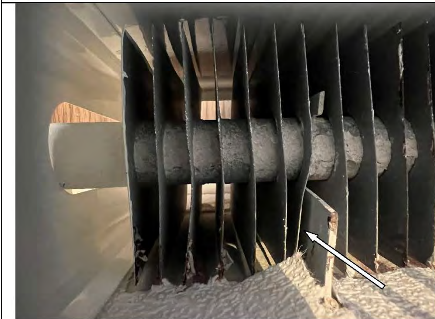
Фото №50. Замытие сот радиатора в кухне.
