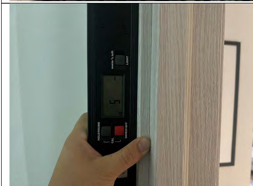
Фото №56. Отклонение наличников дверного блока в ванной комнате по уровню вертикальности составляет 5 мм.
