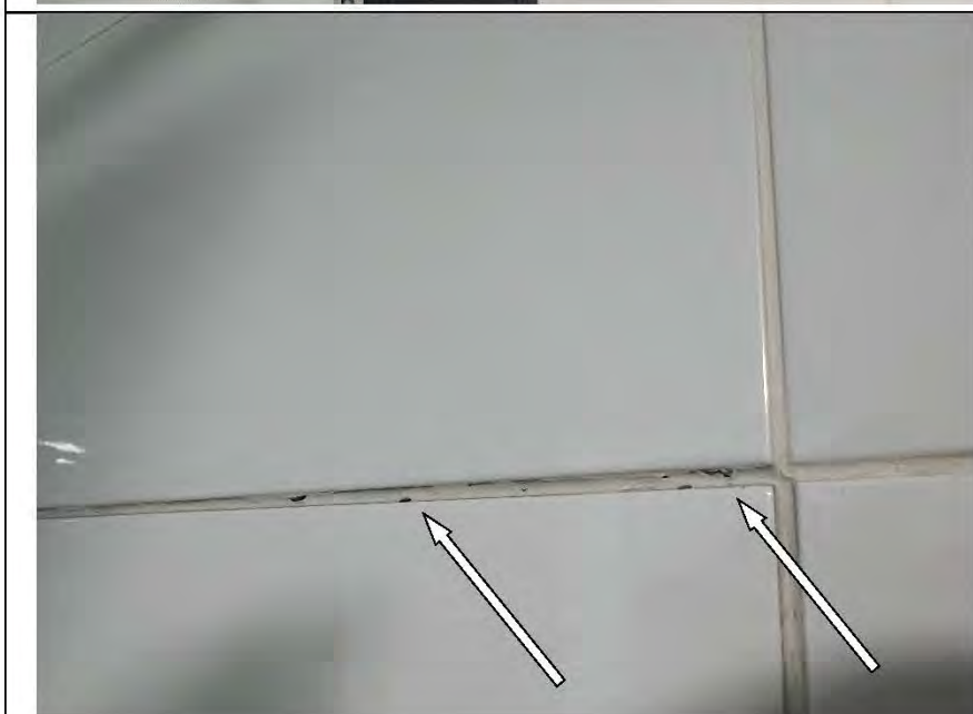
Фото №14. Каверны затирочного раствора в шовном пространстве настенной керамической плитки в ванной комнате.
