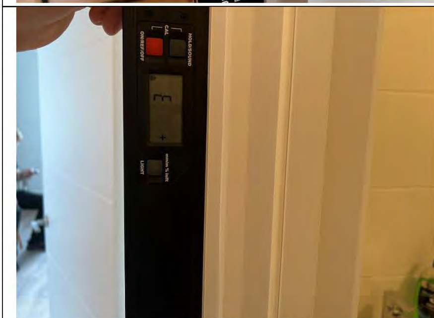
Фото №32. Отклонение от плоскостности и прямолинейности дверного блока в ванной комнате равно 3 мм.
