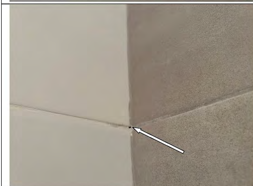
Фото №9. Пропуск затирочного раствора в швах настенной керамической плитки в ванной комнате.
