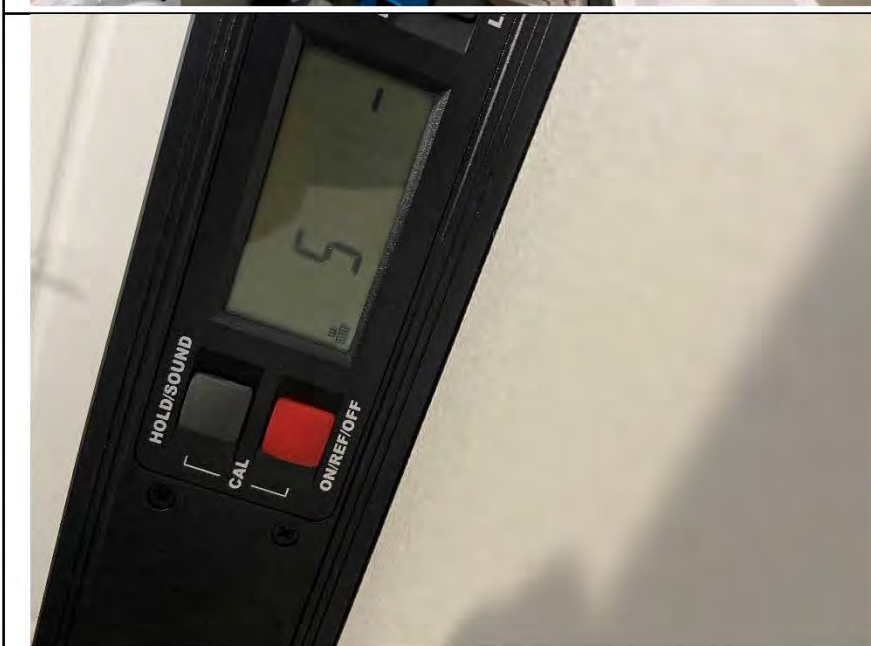
Фото №9. Отклонение поверхности стен от вертикали в коридоре.
