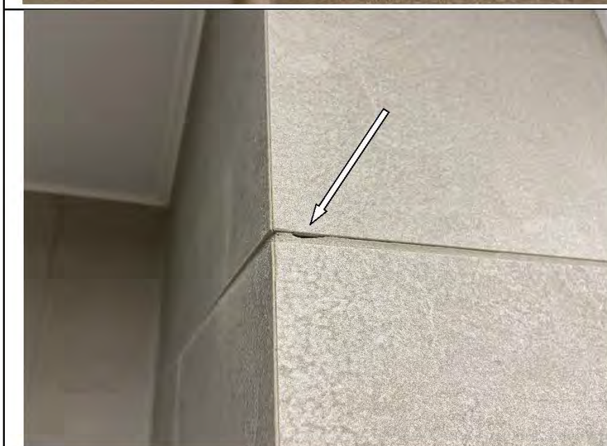
Фото №18. Неровные швы настенной керамической плитки в ванной комнате.
