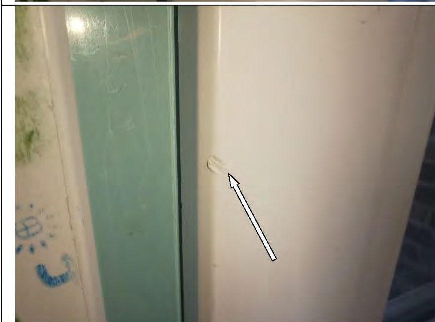
Фото №32. Сколы на профиле ПВХ оконного блока в спальне.
