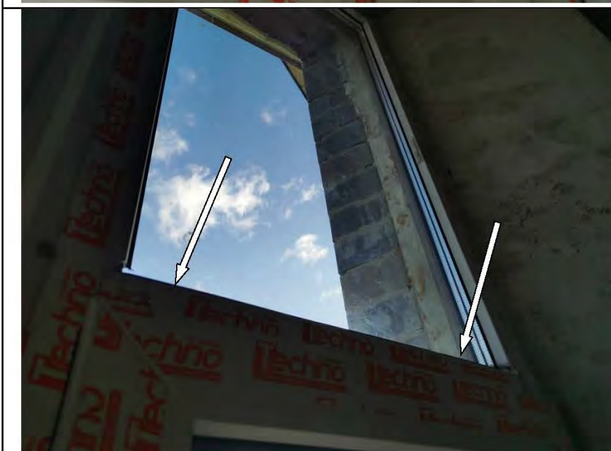
Фото №72. Отсутствует часть штапика на оконном блоке ПВХ в спальне.
