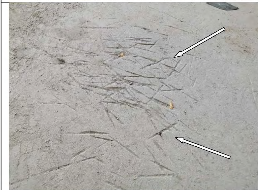
Фото №14. Железобетонные элементы конструкции пола в гостиной имеют дефекты (отсутствие однородности внешнего вида).
