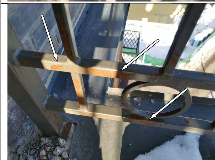
Фото №63. Коррозия на металлическом ограждении оконного блока в гостиной.
