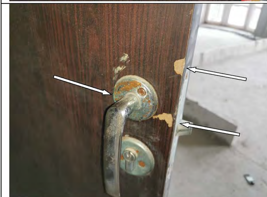
Фото №53. Механические повреждения на лицевой поверхности полотна входного дверного блока. Коррозия на фурнитуре входного дверного блока.
