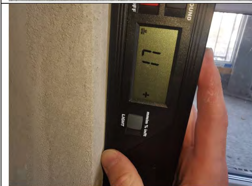
Фото №15. Откос оконного блока в спальне имеет отклонение 17 мм.
