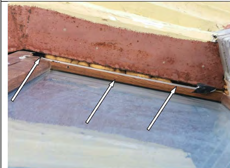
Фото №56. Дефект установки оконного блока ПВХ в спальне (некачественно выполнено заполнение швов монтажной пеной).
