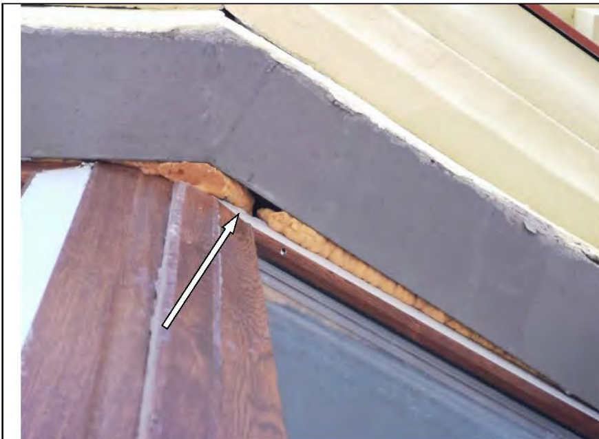
Фото №55. Дефект установки оконного блока ПВХ в гостиной (некачественно выполнено заполнение швов монтажной пеной).
