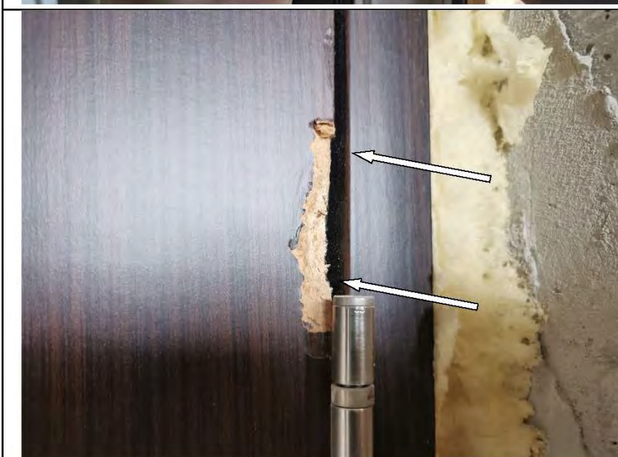
Фото №51. Механические повреждения на лицевой поверхности полотна входного дверного блока.
