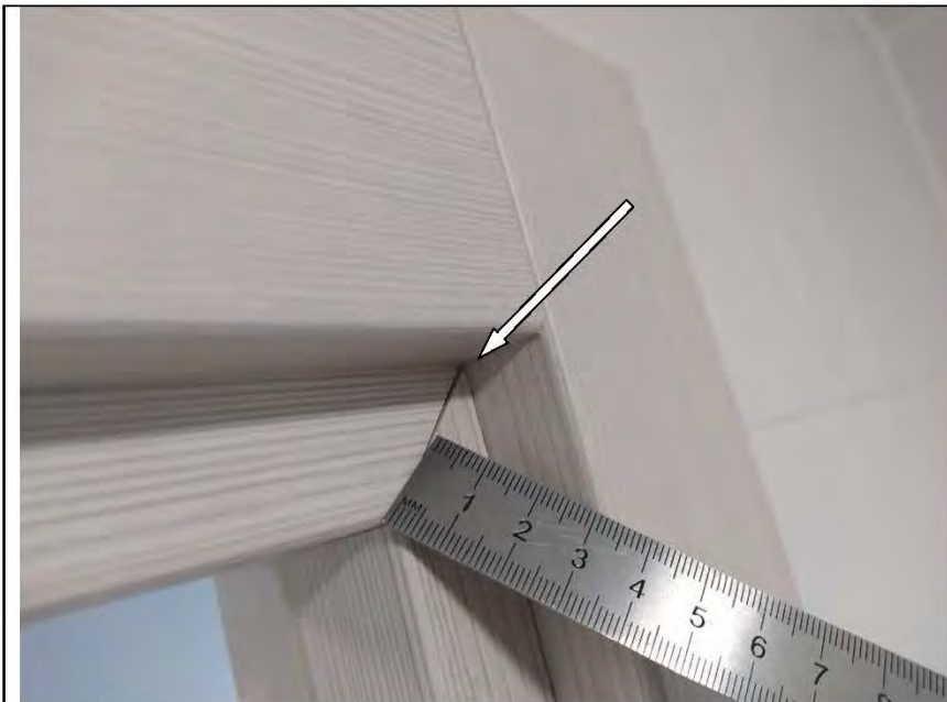
Фото №34. Элементы дверного блока (коробка) соединены не надежно в ванной комнате
