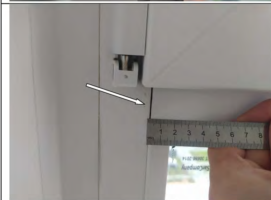
Фото №18. Профиль ПВХ оконного блока в спальне имеет дефекты (зазор).
