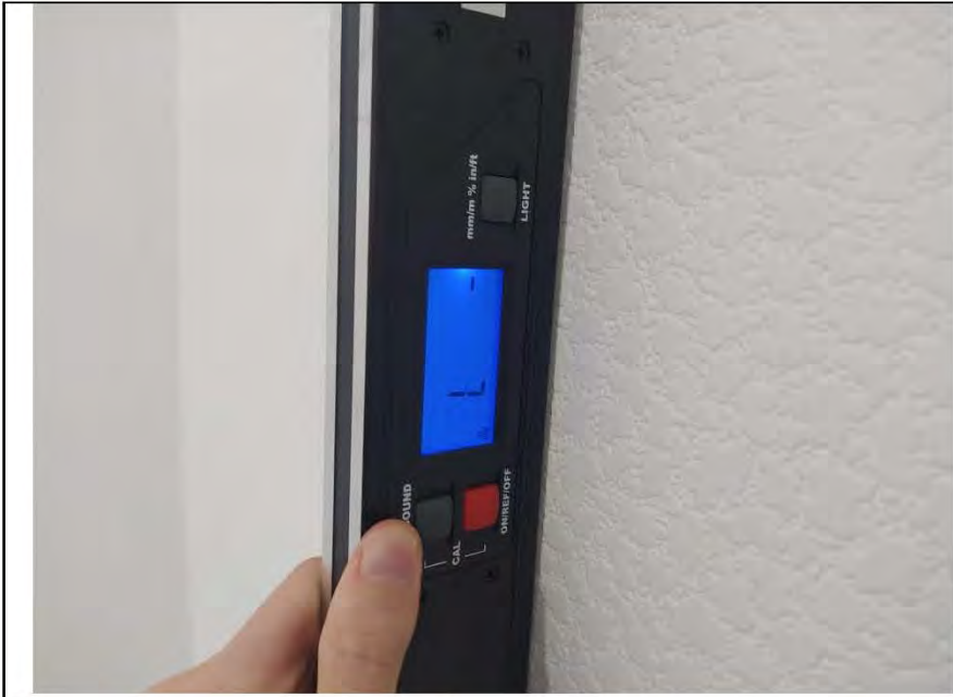
Фото №7. Измерение уровня стен в прихожей.
