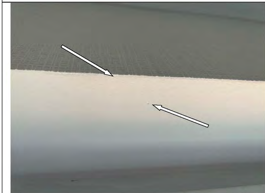
Фото №41. Подтеки краски на откосе оконного блока ПВХ в спальне.
