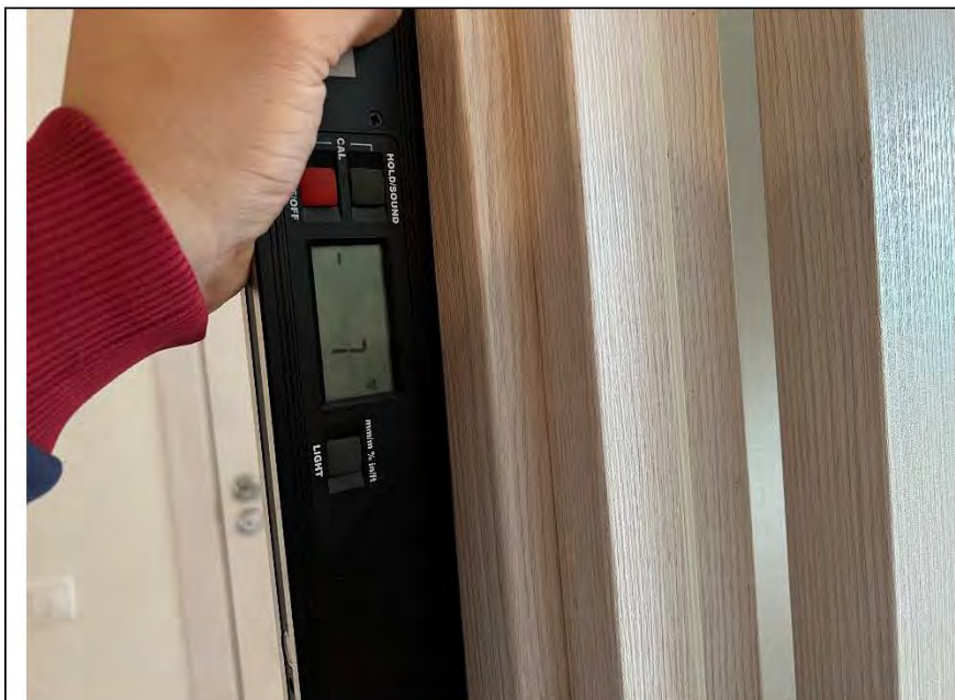
Фото № 70. Отклонение наличников дверного блока в детской равно 7 мм.
