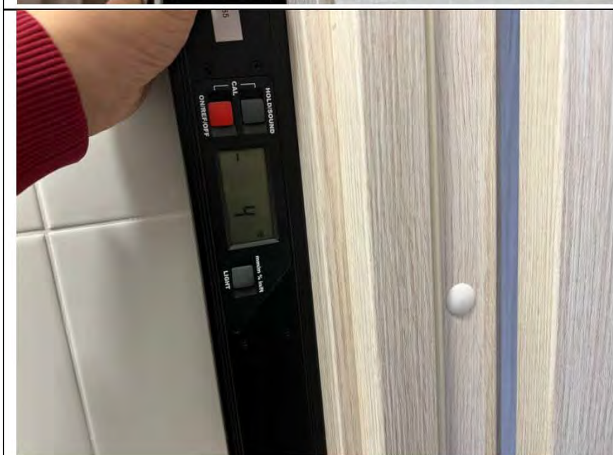
Фото № 72. Отклонение наличников дверного блока в санузле равно 4 мм.
