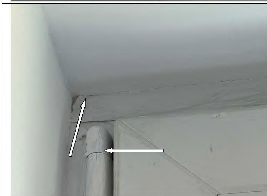
Фото №42. Трещина на откосе оконного блока ПВХ в детской. Загрязнение краской петли оконного блока ПВХ в детской.
