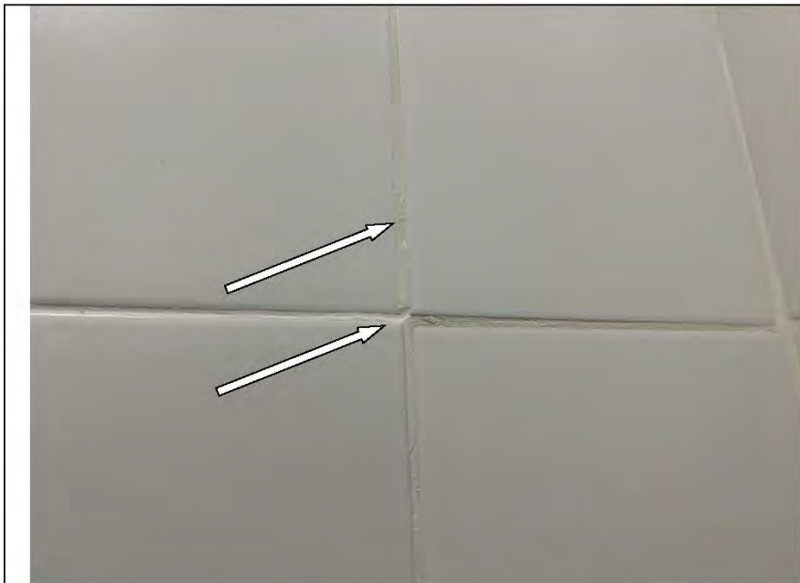
Фото №25. Наплывы затирочного слоя настенной керамической плитки в санузле.
