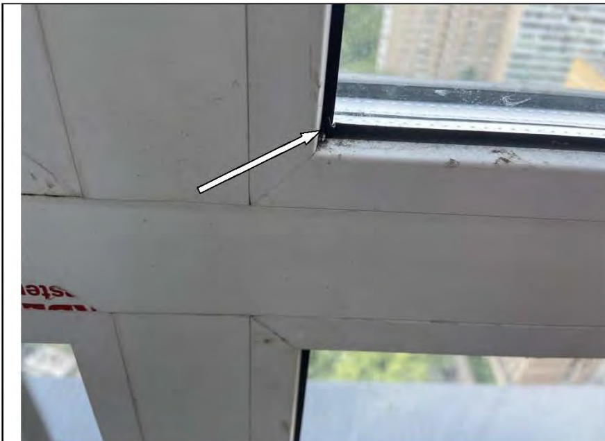
Фото №25. Дефект на уплотнительной ленте оконного блока ПВХ в квартире.
